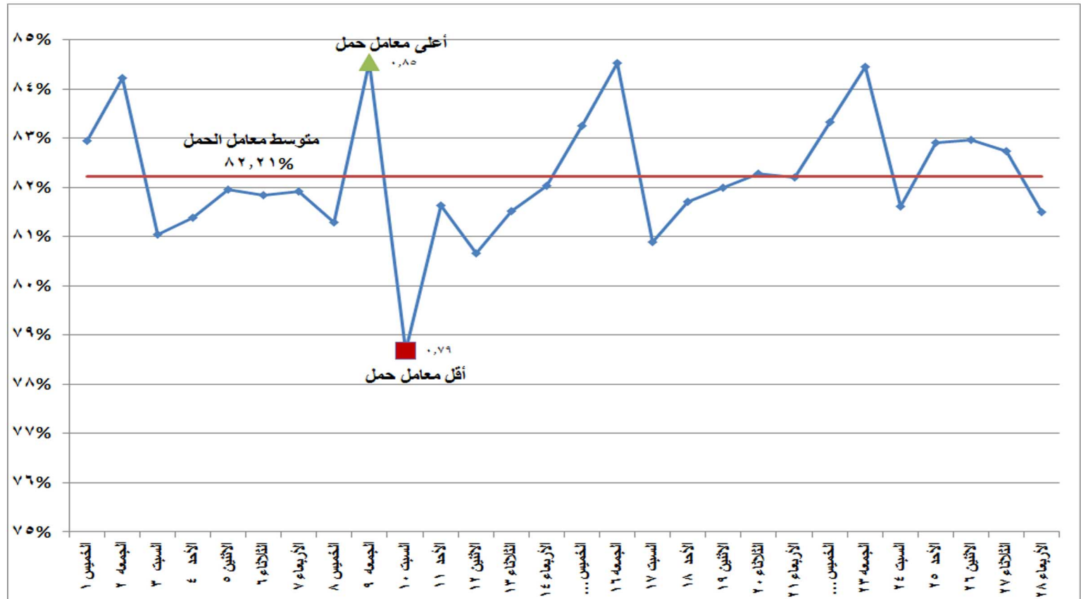
شكل (١٢) إجمالي معامل الحمل لوحدات الانتاج خلال شهر فبراير ٢٠١٨
