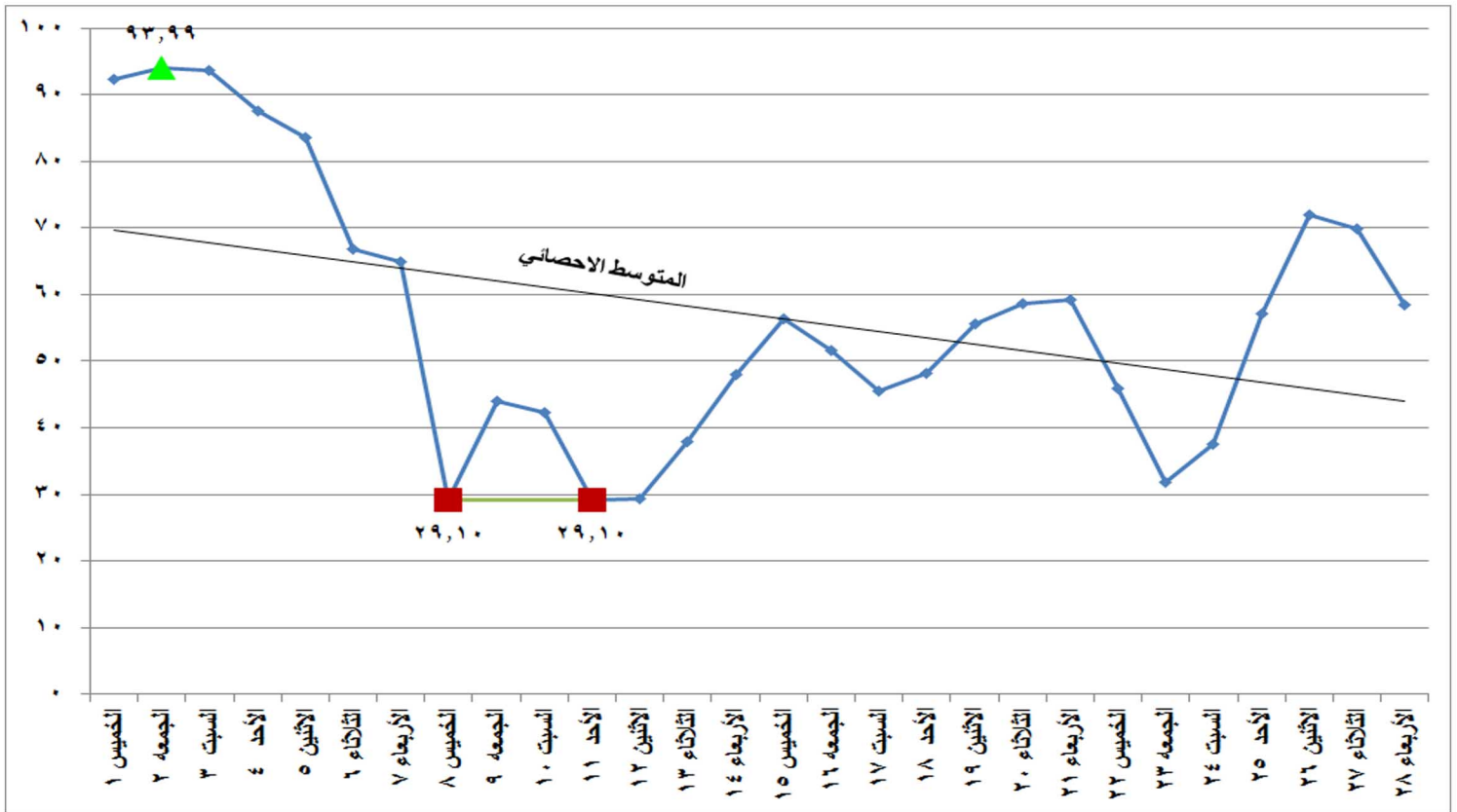
شكل (١٩) الطاقة الكهربائية المنتجة من المازوت خلال شهر فبراير ٢٠١٨
