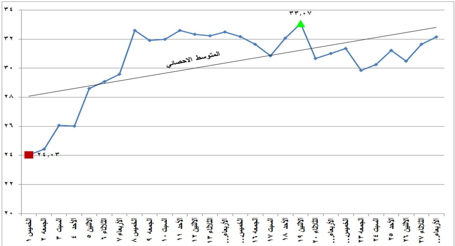
شكل (٢٣) الطاقة الكهربائية المنتجة من المصادر المائية خلال شهر فبراير ٢٠١٨
