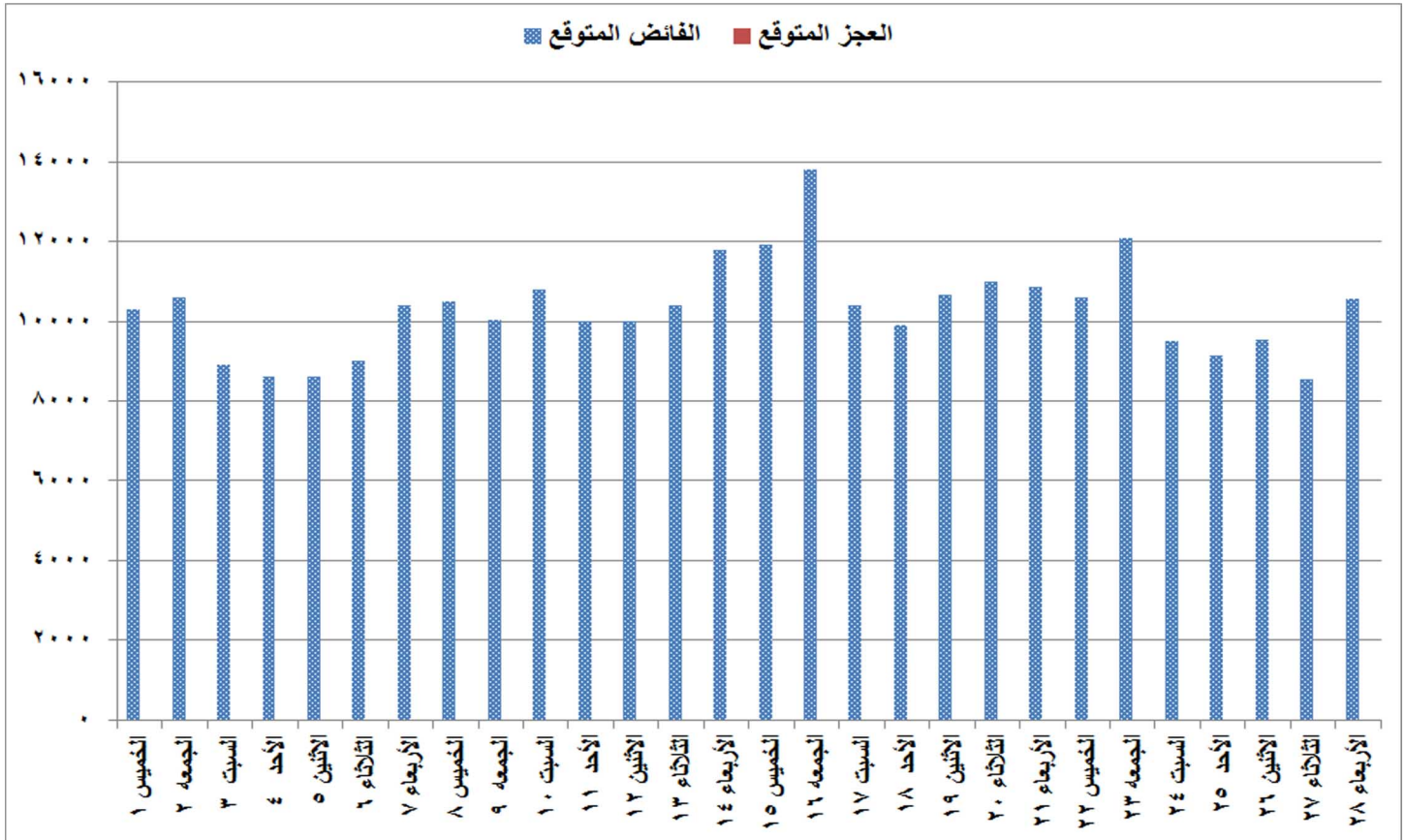
شكل (٧) الفااض والعجز المتوقع للقدرات خلال شهر فبراير ٢٠١٨
