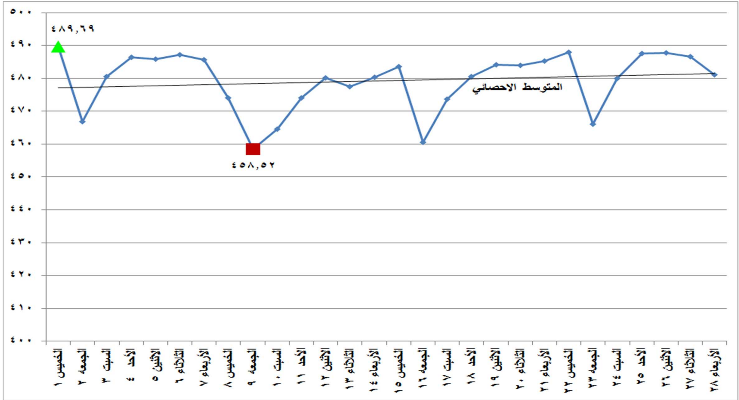
شكل (١٥) إجمالي الطاقة الكهربائية المنتجة من كل المصادر الأولية خلال شهر فبراير ٢٠١٨
