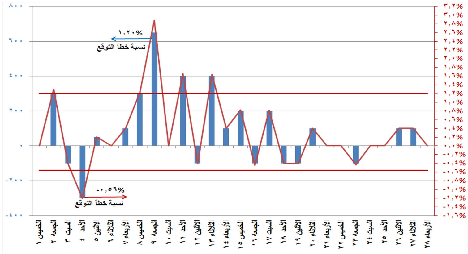
شكل (١٠) الفرق بين الحمل الأقصى المتوقع والمسجل فعليا ونسبة الفرق إلى الحمل المسجل فعليا خلال شهر فبراير ٢٠١٨
