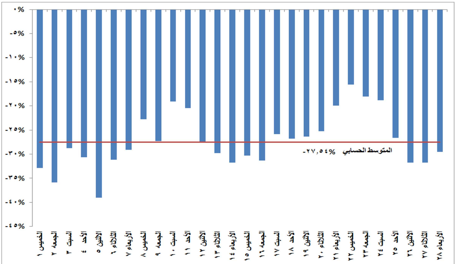
شكل (١٨) نسب التغير في استخدام الغاز الطبيعي في إنتاج الطاقة الكهربائية خلال شهر فبراير ٢٠١٨ مقارنة بالشهر المماثل من العام السابق
