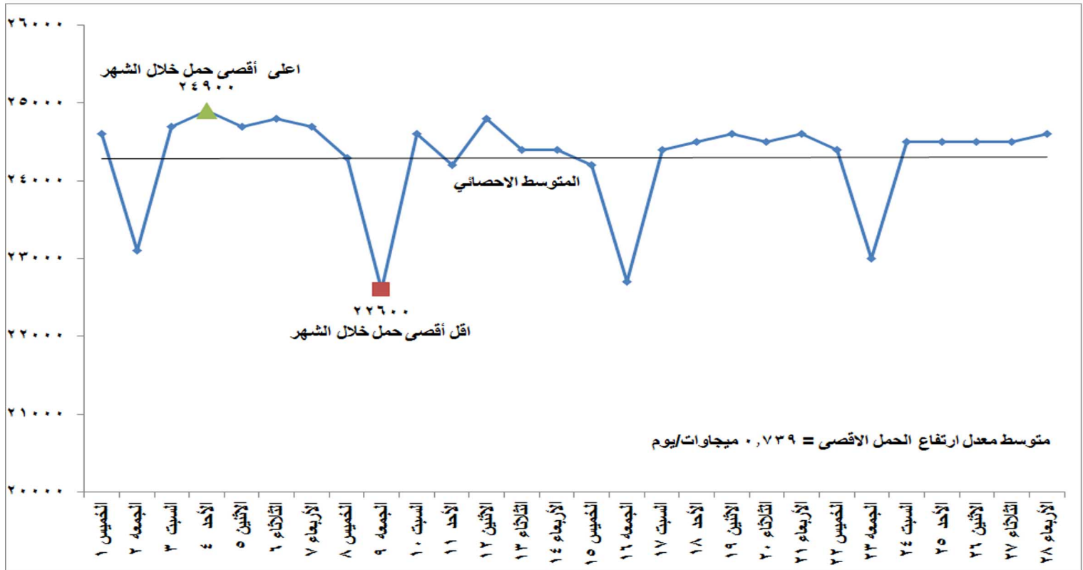
شكل (١) تطور الحمل الاقصى اليومي خلال شهر فبراير ٢٠١٨
