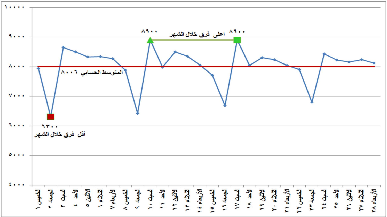
شكل (٣) الفرق بين أقصى وأدنى حمل خلال شهر فبراير ٢٠١٨
