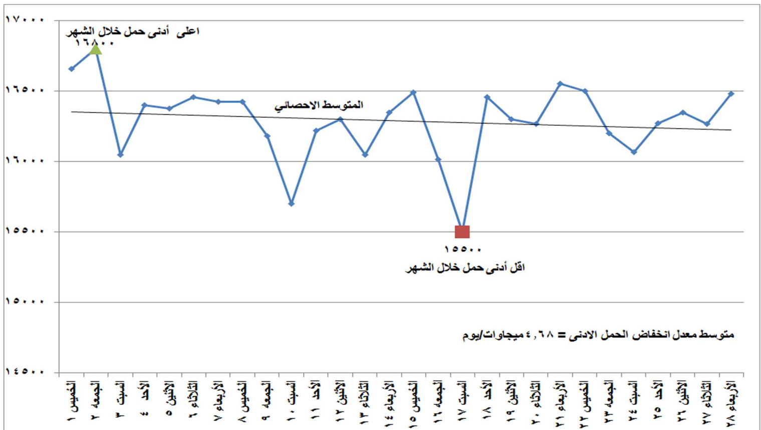
شكل (٢) تطور الحمل الادنى اليومي خلال شهر فبراير ٢٠١٨
