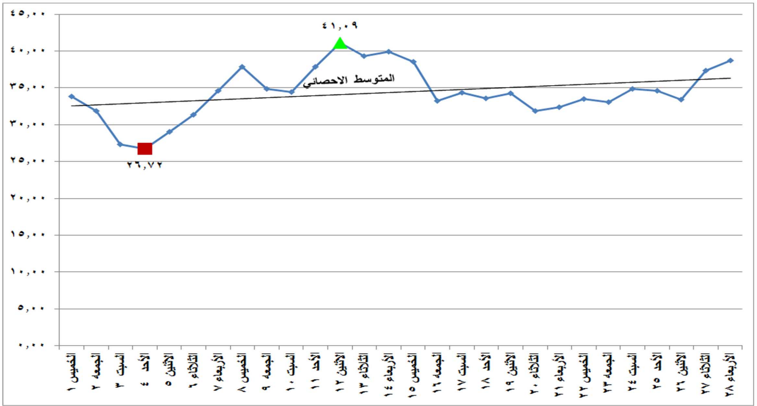
شكل (٢١) الطاقة الكهربائية المنتجة من المصادر غير الحرارية خلال شهر فبراير ٢٠١٨
