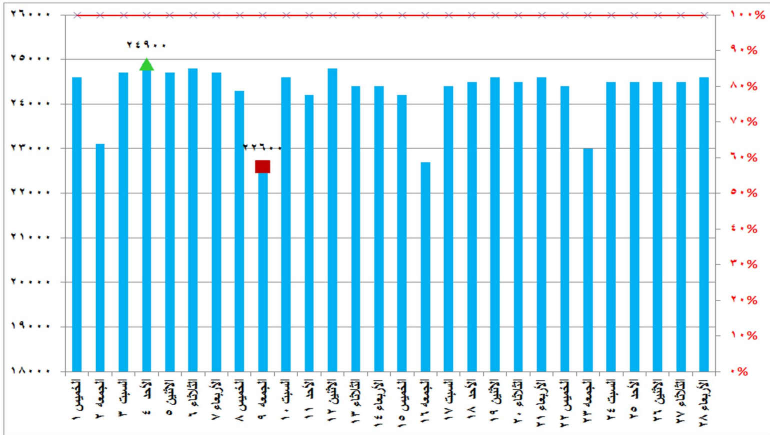
شكل (٥) قدرات الانتاج المتاحة ونسبتها للحمل الأقصى خلال شهر فبراير ٢٠١٨
