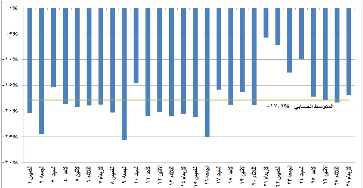
شكل (٩) النسب المئوية للتغير في الحمل الاقصى خلال شهر فبراير ٢٠١٨ مقارنة باليوم المماثل من العام الماضي
